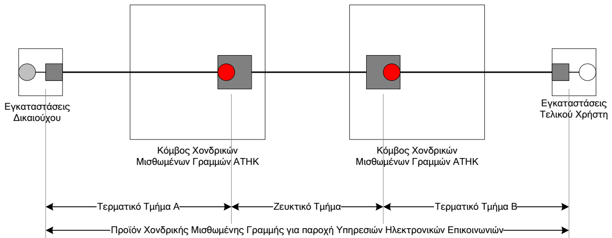
Σχήμα 2.1: Προϊόν Χονδρικής Μισθωμένης Γραμμής
