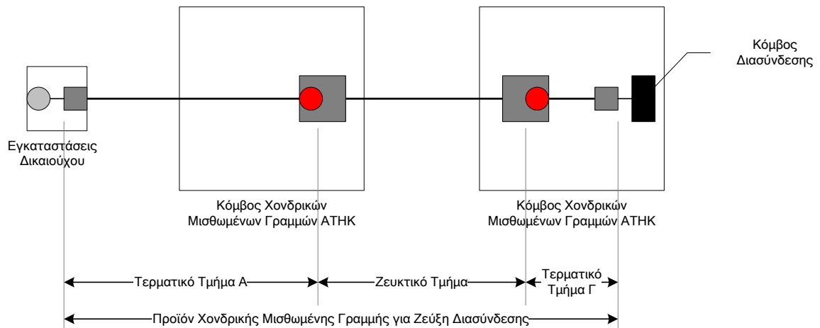
Σχήμα 2.1: Προϊόν Χονδρικής Μισθωμένης Γραμμής για Ζεύξη Διασύνδεσης με χρήση Τερματικού Τμήματος Α.
