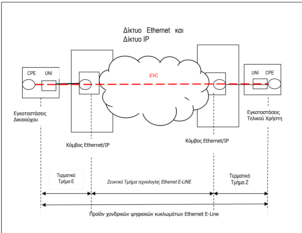
Σχήμα 3.1: Προϊόν Χονδρικών Ψηφιακών Κυκλωμάτων Ethernet E-line
