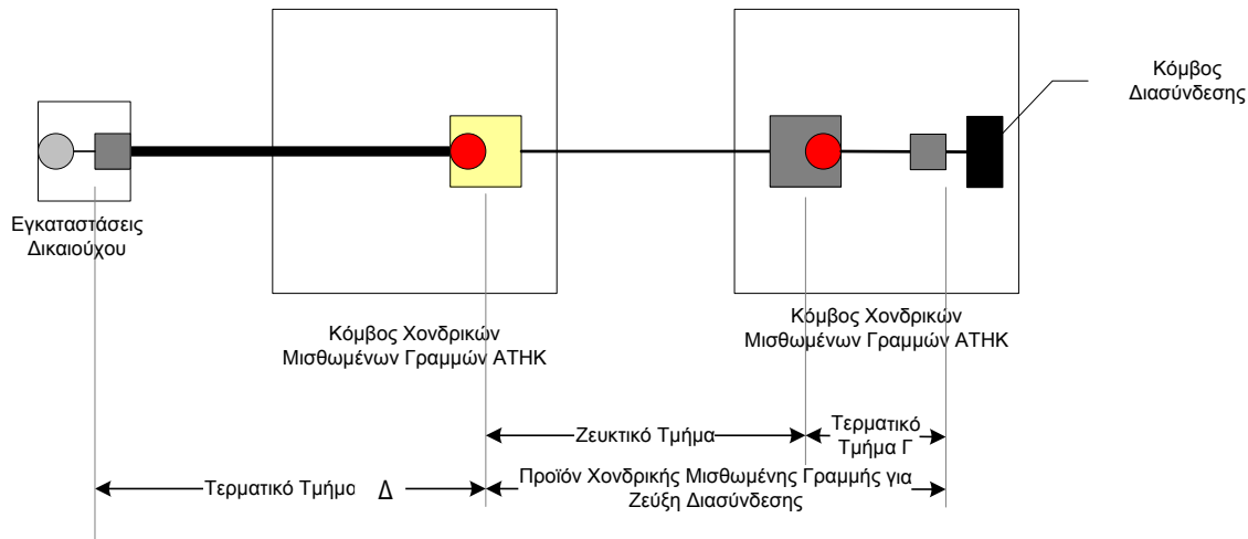
Σχήμα 2.2 : Προϊόν Χονδρικής Μισθωμένης Γραμμής για Ζεύξη Διασύνδεσης με χρήση Τερματικού Τμήματος Δ.
