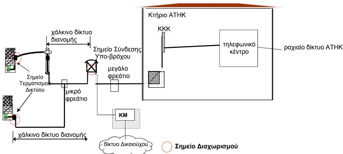
Σχ. 1-4: Πλήρως Αδεσμοποίητη Πρόσβαση στον Τοπικό Υπο-βρόχο
