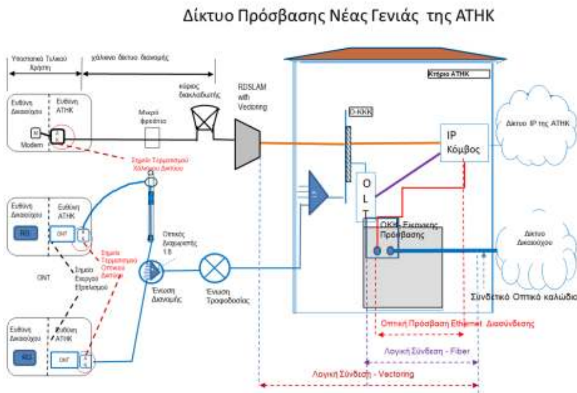
Σχ. 1-6: Σύνδεση στον Τοπικό Κόμβο IP του Δικτύου Νέας Γενιάς (NGN) της ΑΤΗΚ
