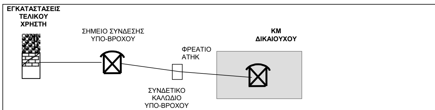
Σχεδιάγραμμα 2-5 Συνεγκατάσταση στο Σημείο Σύνδεσης Υπο-βρόχου
